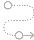
Letzte Meile
